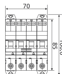
4 POLE , SPN
